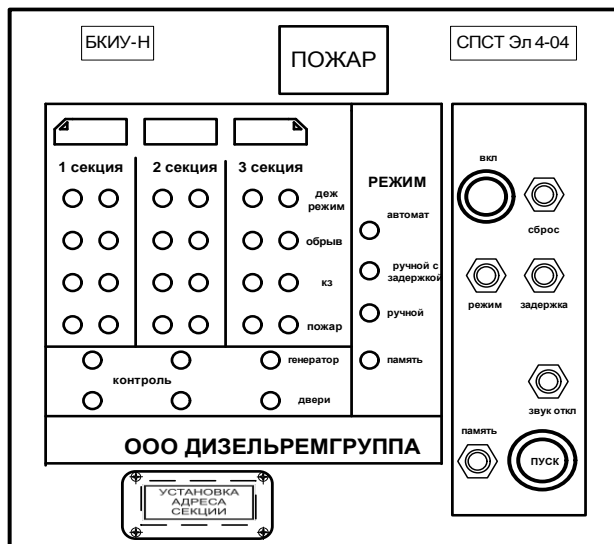
Рис.1.1 Расположение органов управления и элементов индикации БКИУ
