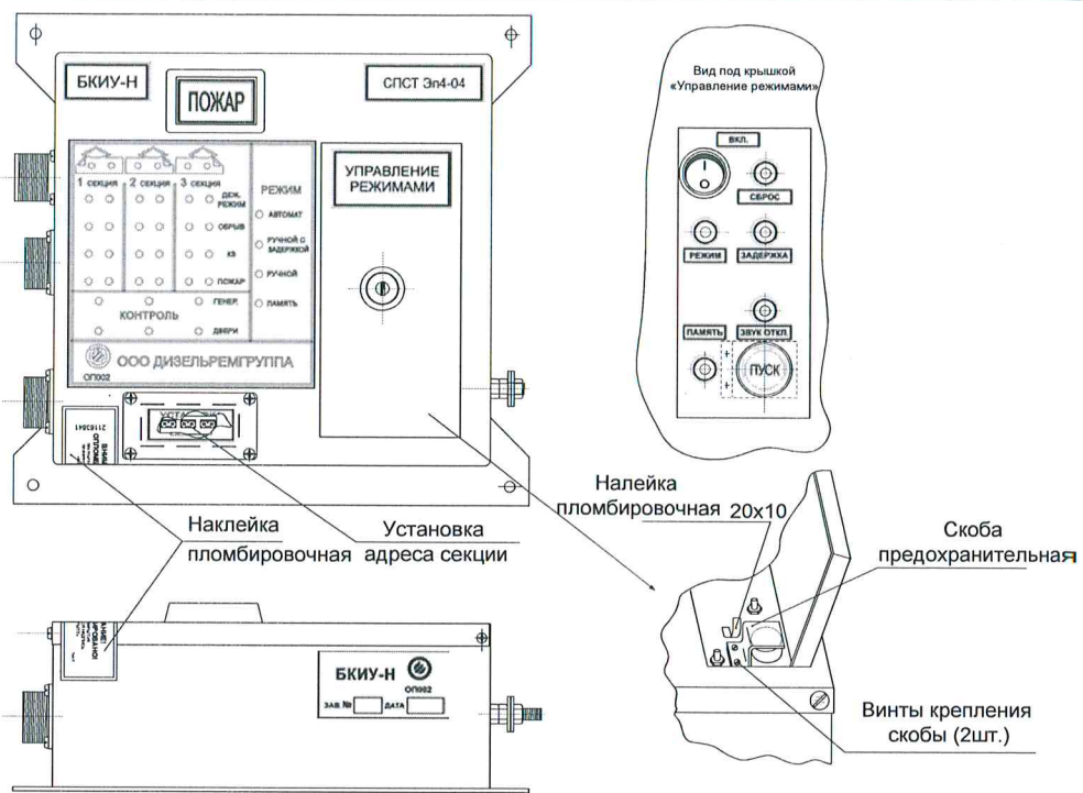
Рис.13.2 - Пломбирование блока БКИУ
