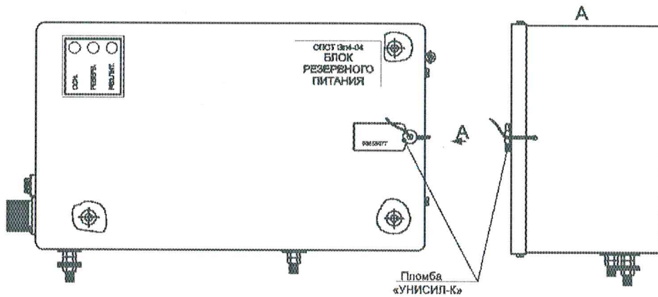
Рис.13.3 - Пломбирование блока БРП
